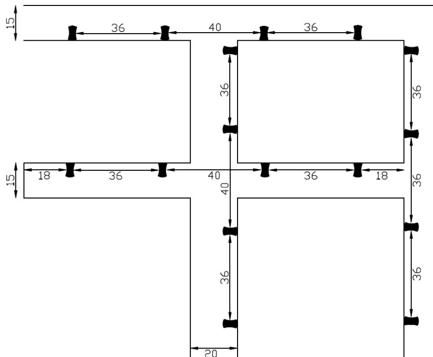
Figura 2 - Distâncias máximas permitidas entre postes com iluminação.
